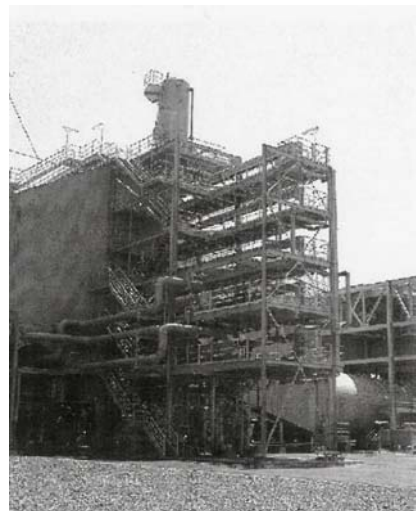
排ガス加熱器(再加熱)製作据付工事
