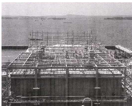
脱硫晶析槽製作据付工事
